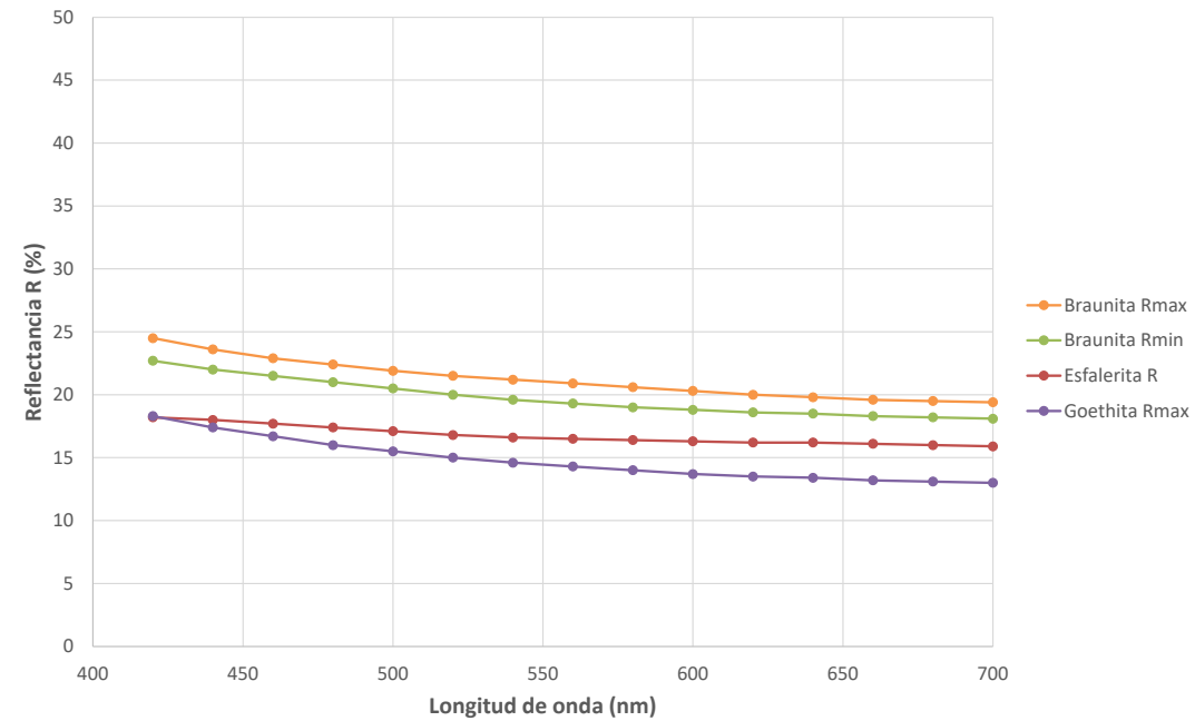
Reflectancia especular en el espectro visible en Picot&Johan (1982) de Braunita Rmax, Braunita Rmin, Esfalerita R y Goethita Rmax
