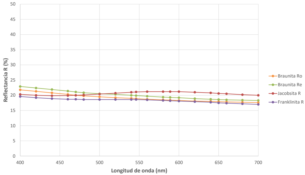
Reflectancia especular en el espectro visible en QDF3 de Braunita Ro, Braunita Re, Jacobsita R y Franklinita R
