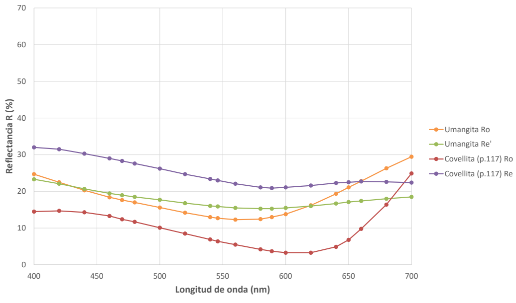
Reflectancia especular en el espectro visible en QDF3 de Umangita Ro, Umangita Re', Covellita (p.117) Ro y Covellita (p.117) Re
