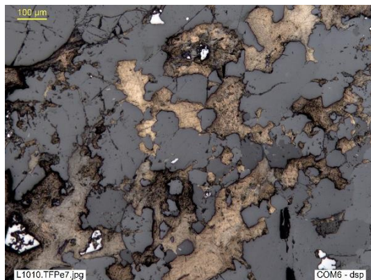
F COM6 y F COM7 (Misma escena, dsp y d+p , resp ). Carbonatita (calcita, gris, anisótropa) con magnetita diseminada (blanca, isótropa) y valleriita (gris claro a pardo grisáceo, birreflectante, pleocroica y fuertemente anisótropa, parecida al grafito pero no tan birreflectante como éste). TFPe7, Palabora (Rep. Surafricana).
