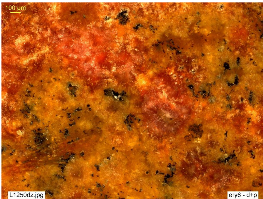
F ery5 y F ery6 (Misma escena: osp y o+p, resp). Agregados fibroso-radiados, intercrecidos, de oro pimente (gris claro, RI amarillas) y eritrina (gris más oscuro, RI rosadas), con escasos relictos de arseniuro (puntos blancos, brillantes, posible safflorita). CR375, Cobalt, Ontario, Canadá.
