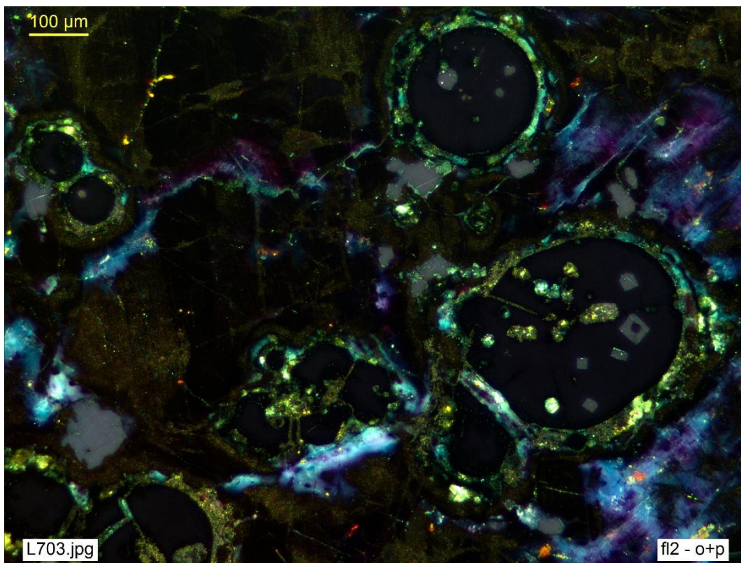
F fl1 y F fl2 (Misma escena: dsp y o+p , resp). Mena de fluorita (gris oscuro) y uraninita (gris: esferoides rodeados de corona de alteración con diminutos corpúsculos de pirita, amarilla), con inclusiones de galena (blanca). En F fl2 ( o+p ), todos ellos están en extinción (minerales cúbicos): se ve únicamente una luminosidad difusa, por las reflexiones internas de fluorita (violáceas) y del halo de alteración de uraninita. HD6023, Wolsendorf, Baviera, Alemania.
