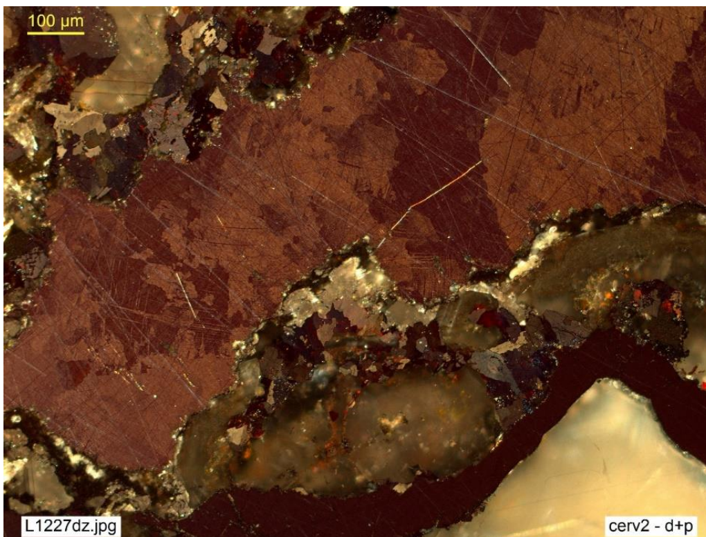
F cerv1 y F cerv2 (Misma escena: dsp y d+p , resp). Mena argentífera antimonial: masa de Sb (centro: blanco muy brillante, anisótropo), parcialmente alterado a cervantita cerv (zonas marginales: gris oscuro, fibroso, abundantes RI incoloras), con orla de pirargirita prg (gris azulado, RI rojas, anisótropo) y corona externa de galena gn (banda inf dch: blanco grisáceo, isotropa). La gg de q y Carb , gris muy oscuro, se caracteriza ( d+p ) por las abundantes RI incoloras de ambos y por las maclas de Carb . CR398, Hiendelaencina, Guadalajara.
